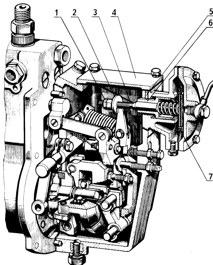
1 - контргайка; 2 - упор; 3 - штифт; 4 - крышка; 5 - штифт; 6 - втулка; 7 - диафрагма. Рисунок 27 - Регулировка топливного насоса с противодымным корректором.
