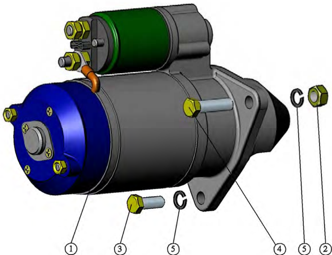
Рис. 17 Установка стартера.
