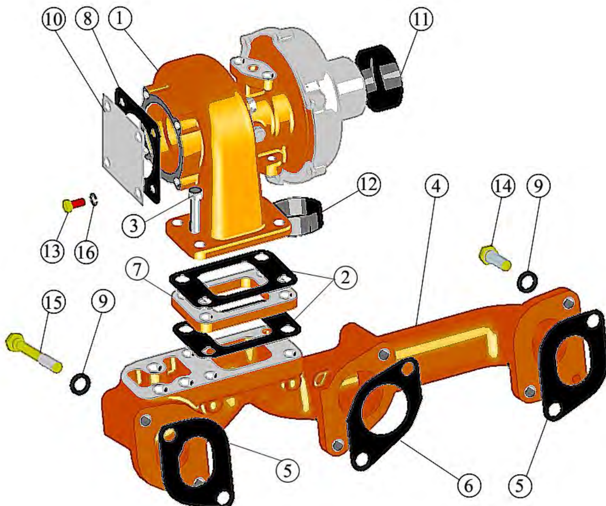
Рис. 6 Установка турбокомпрессора.
