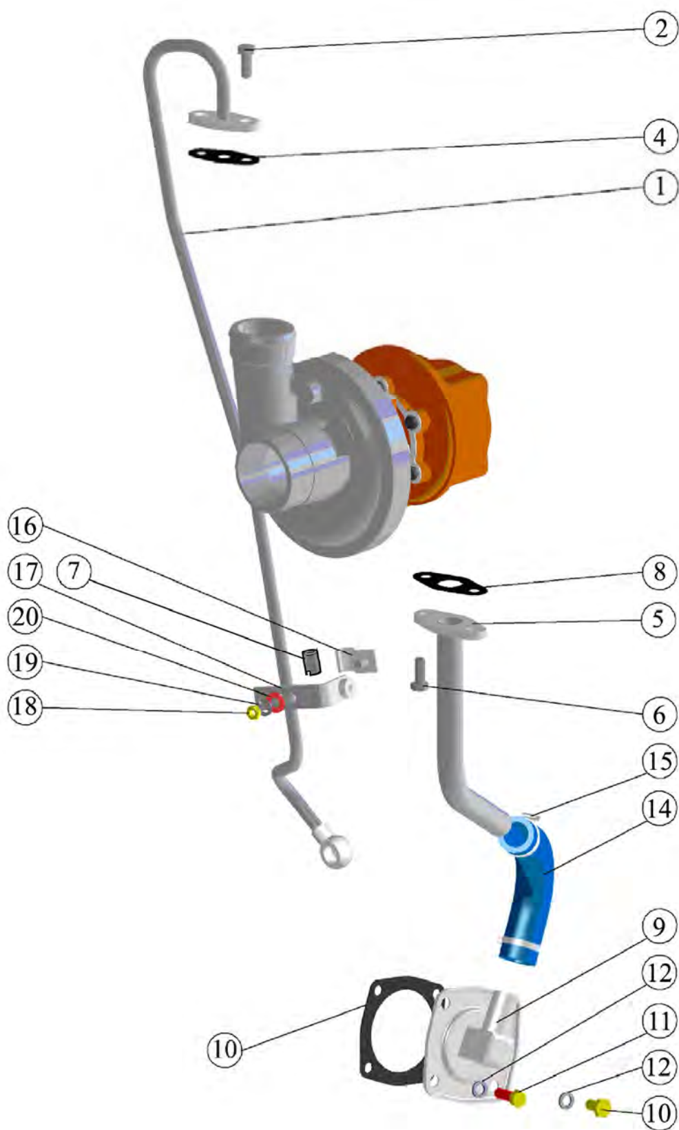
Рис. 15 Маслопроводы турбокомпрессора.
